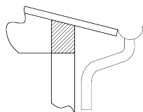
PARTICOLARE CANALE DI GRONDA
